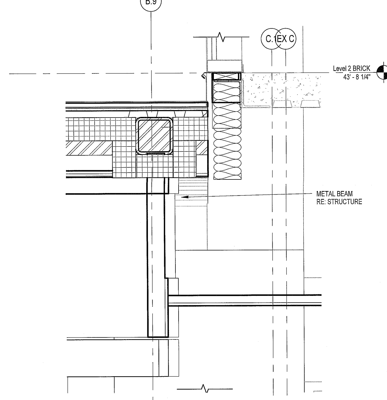
D2 CANOPY SECTION - FLASHING SCALE: 1" = 1'-0"
