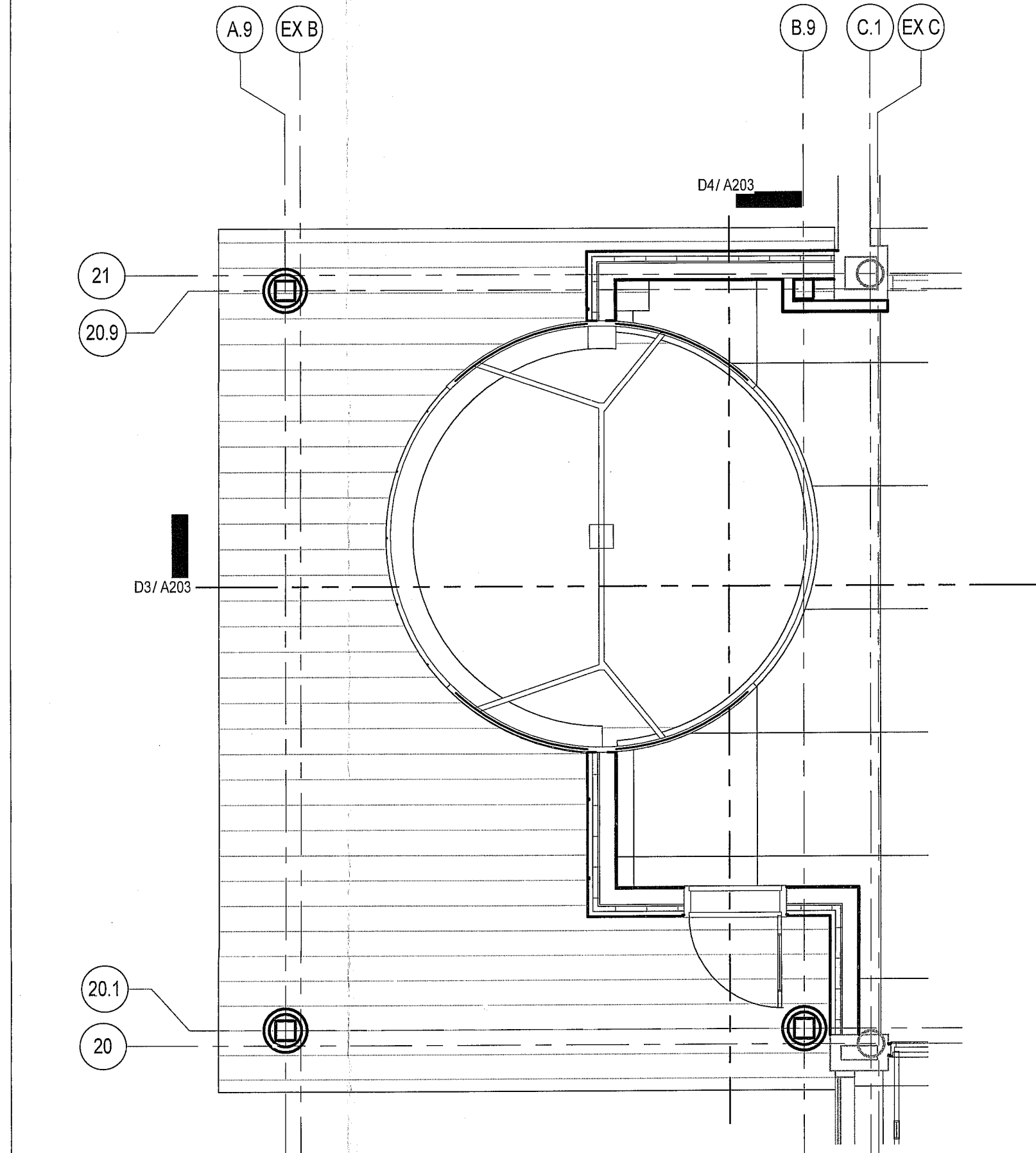
A3 CANOPY SOFFIT/CEILING PLAN SCALE: 1/4" = 1'-0"
