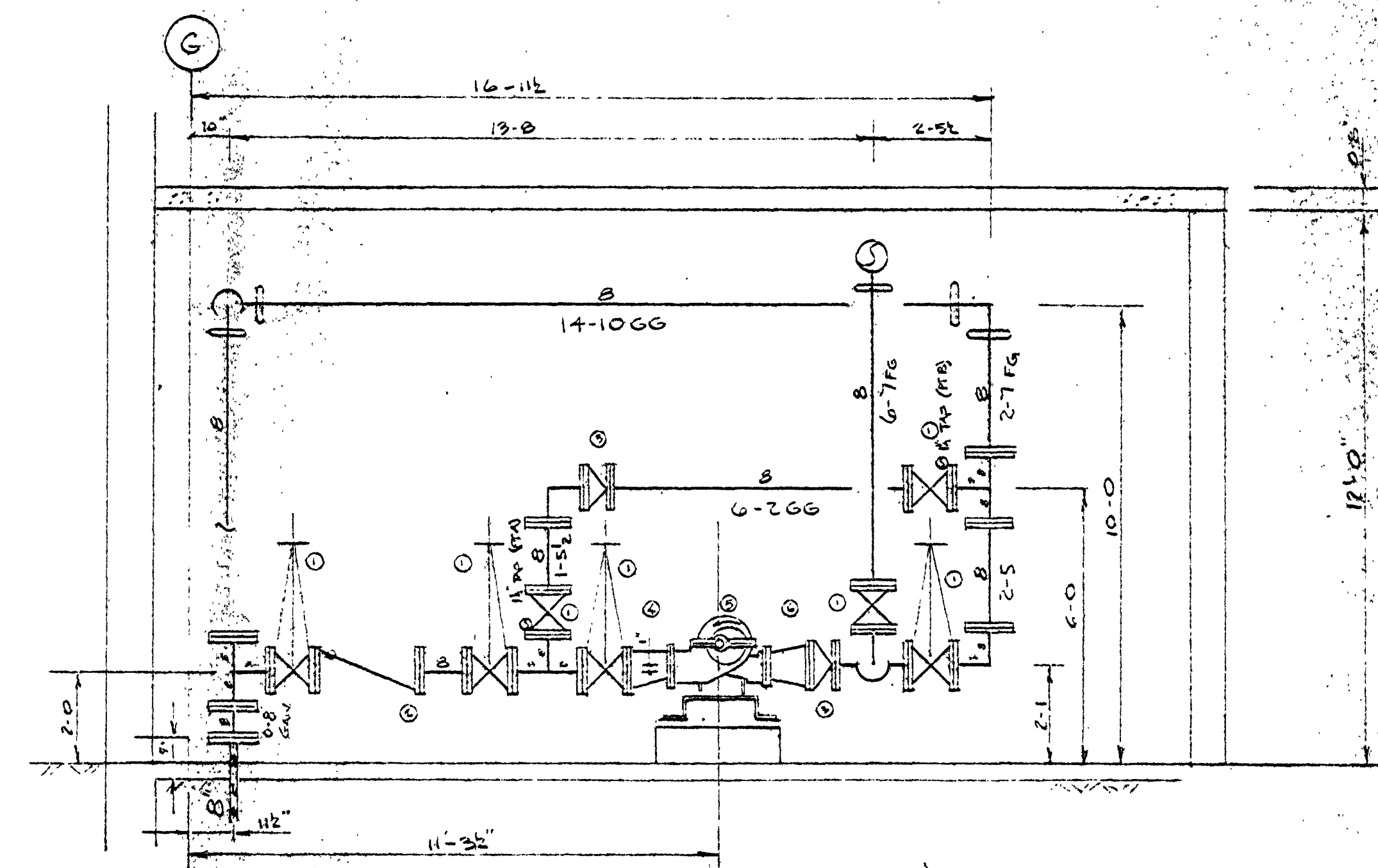
SECTION A-A 1/8" = 1'-0"
